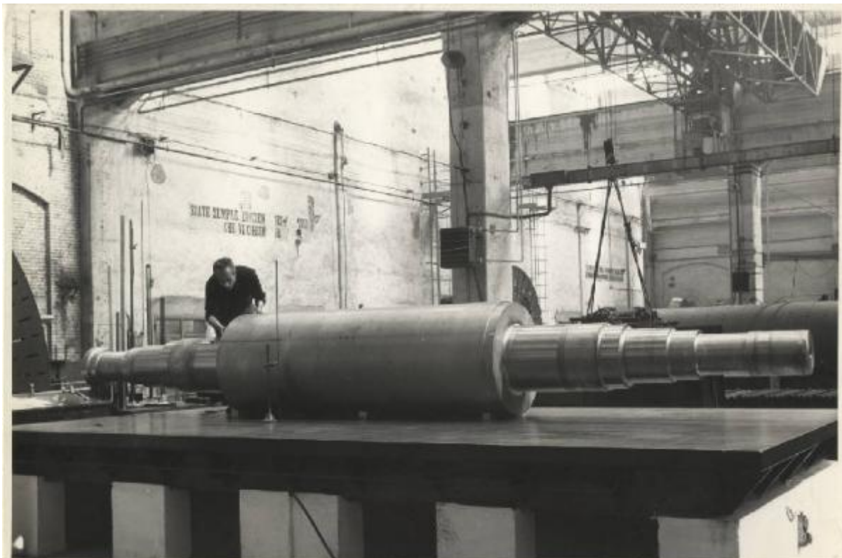
8754/939 - Turboalternatore sincrono trifase (con raffreddamento ad aria in ciclo chiuso) 30.000 kVA - 10.500 V - 50 Hz - 3.000 g/l' per E.N.E.L. - Compartimento di Firenze - C.le di Castelnuovo
